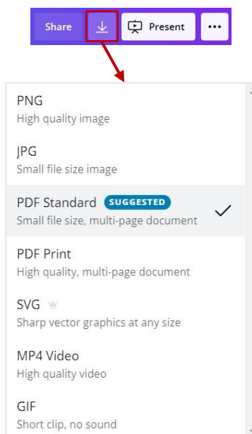
Figura 7. Descărcarea prezentării
