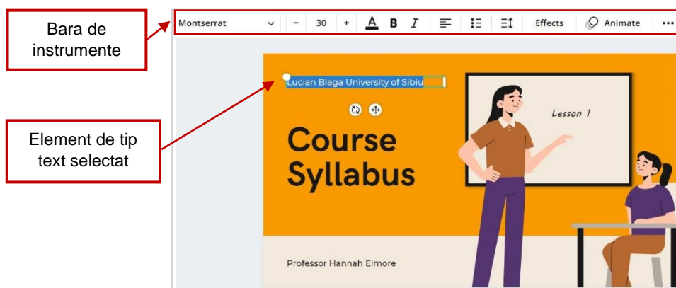
Figura 5. Editarea/formatarea elementelor
