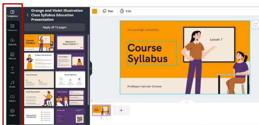
Figura 6. Elemente suplimentare
